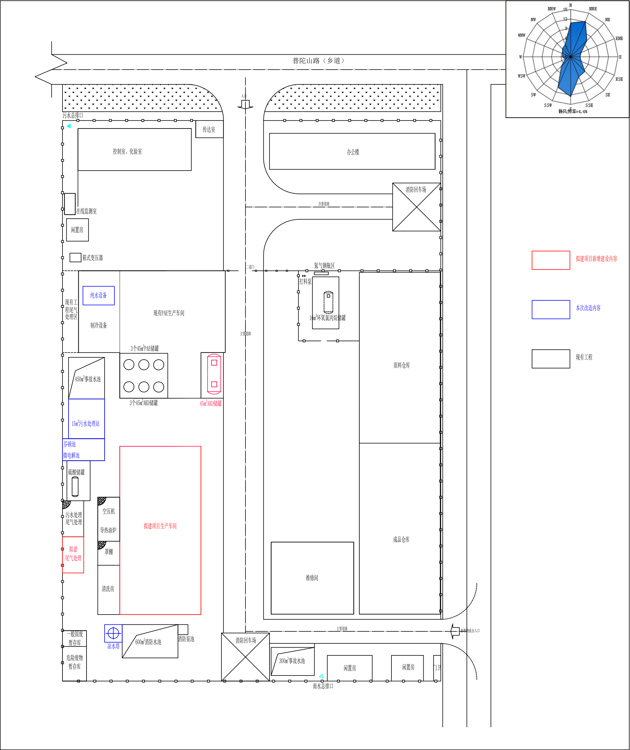
图3-1 拟建项目建成后全厂总平面布置图 比例尺 1:1000
