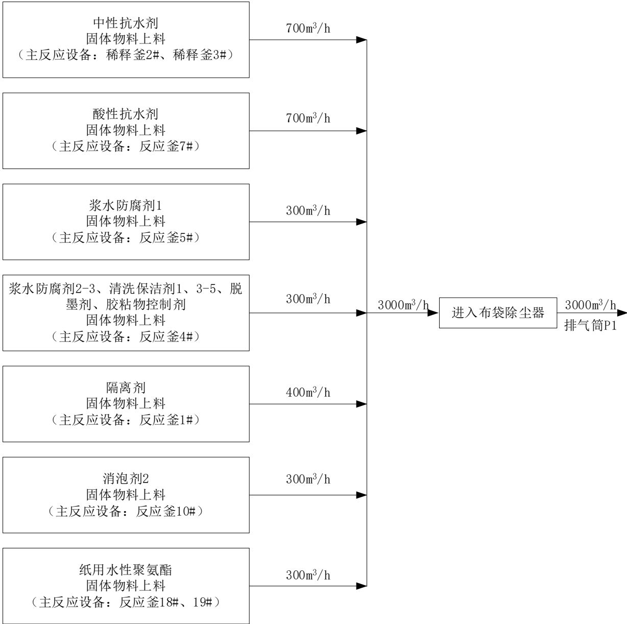
图 3-10 拟建项目风量配置示意图 (排气筒 P1)
