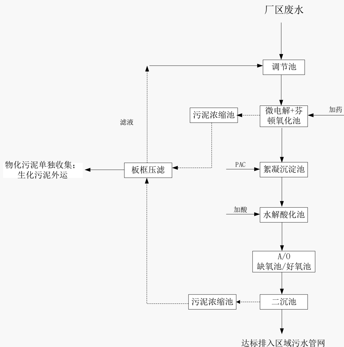
图 2-8 厂区 10\text{m}^3/\text{d} 污水处理站工艺流程图
