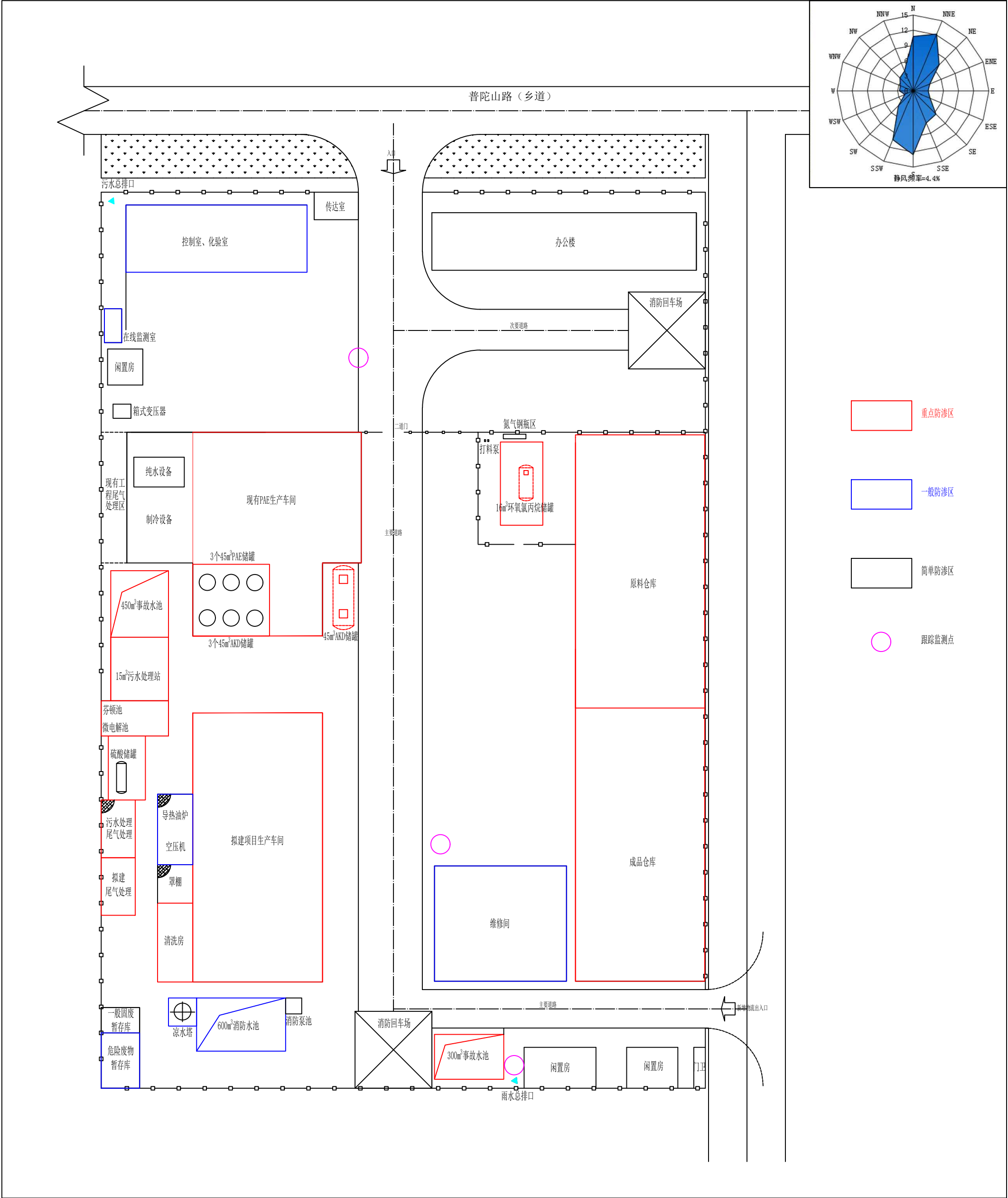
图5-17 全厂分区防渗图 比例尺 1:1000
