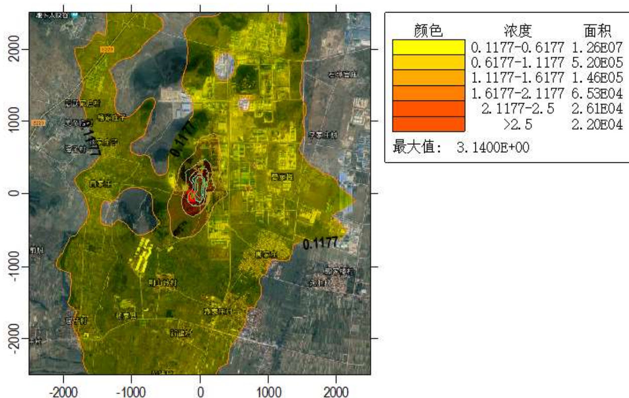
图 5-7 各网格点 PM_{2.5} 叠加背景值后 95%保证率日最大平均浓度分布图 单位: \mu g/m^3
