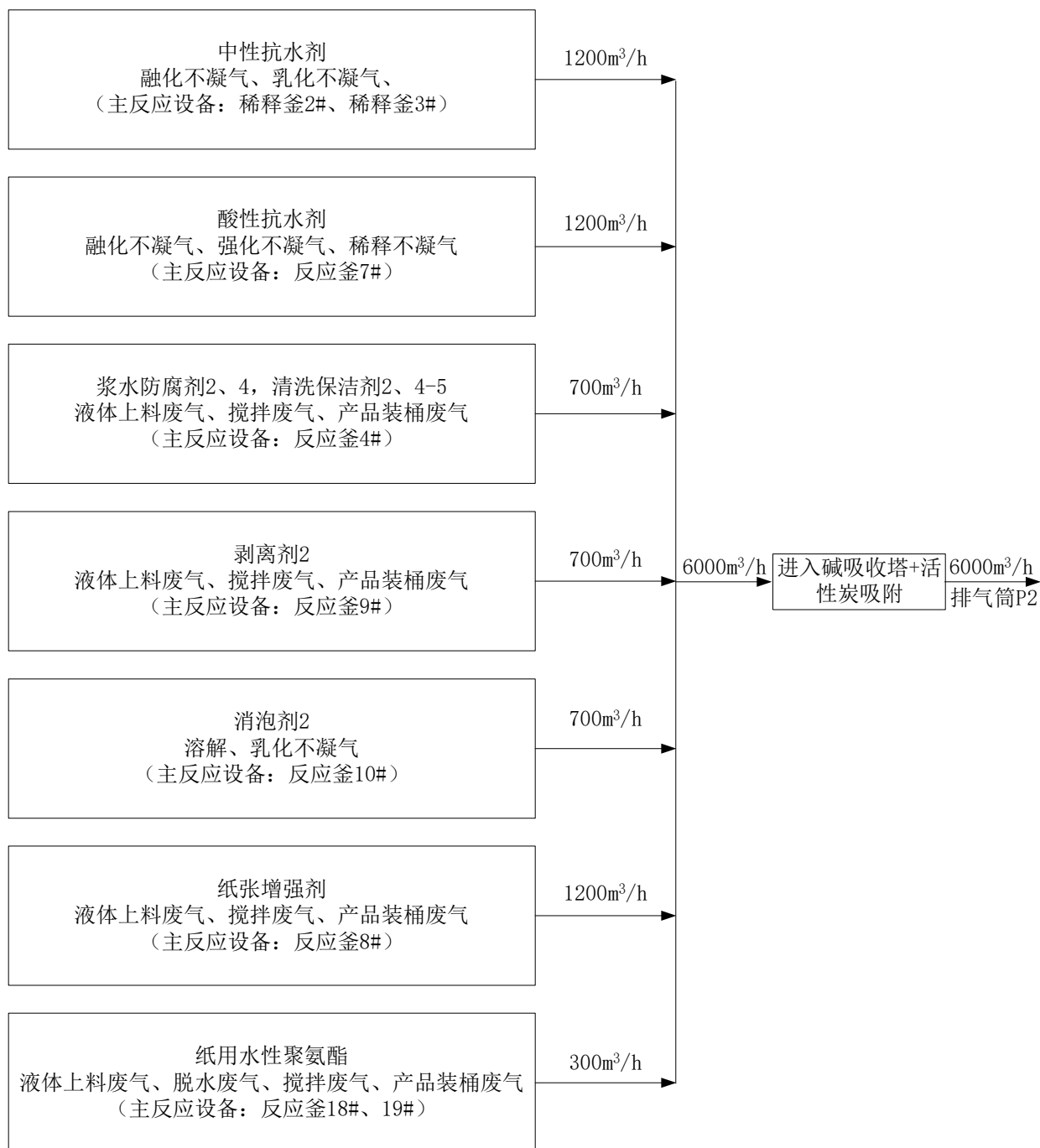
图 3-11 拟建项目风量配置示意图（排气筒 P2）
