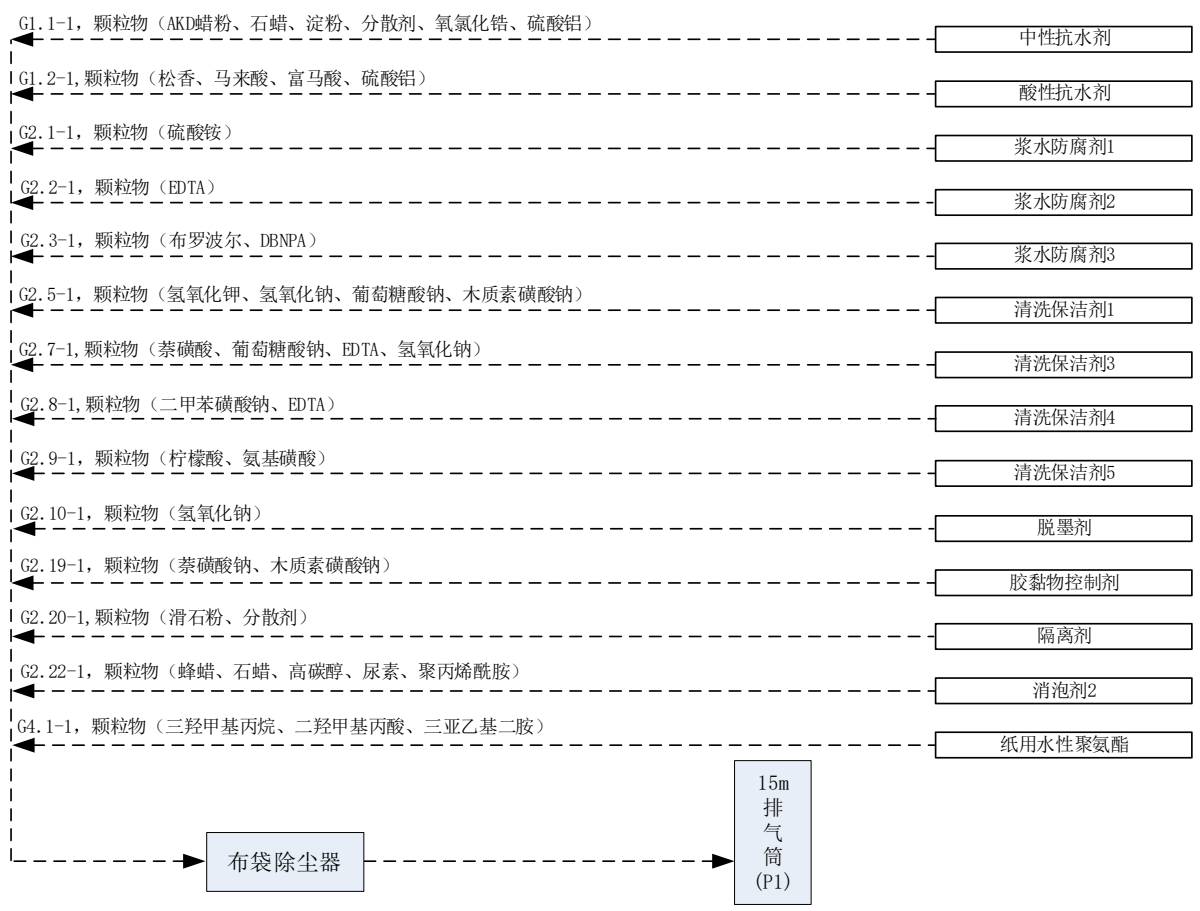
图 3-8 拟建项目工艺有组织废气处理系统示意图（排气筒 P1）
