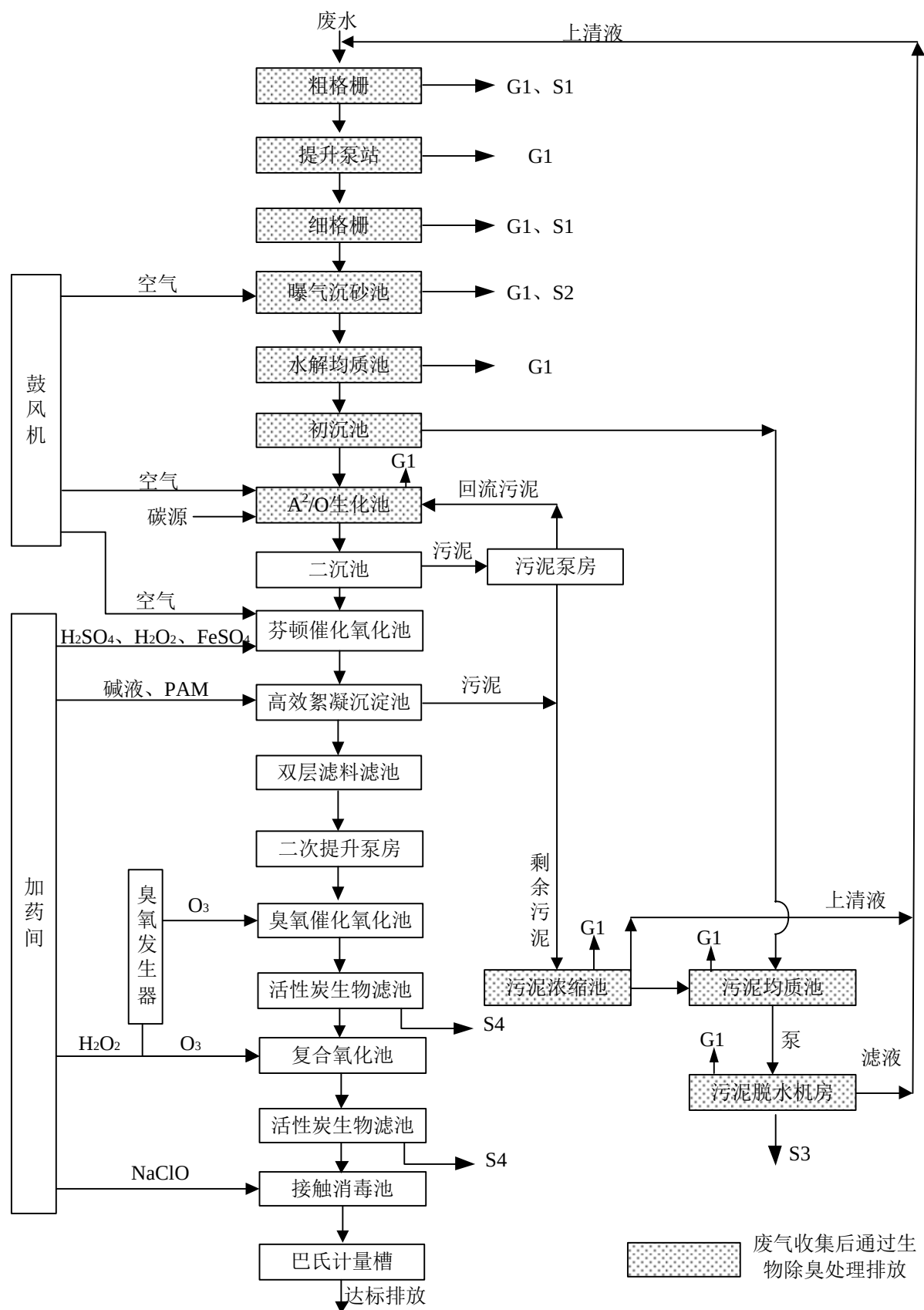
图 5-9 沂水城投庐山水务有限公司污水处理工艺流程图
