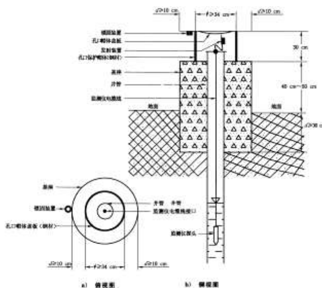
图 5-18 孔口保护装置结构示意图
