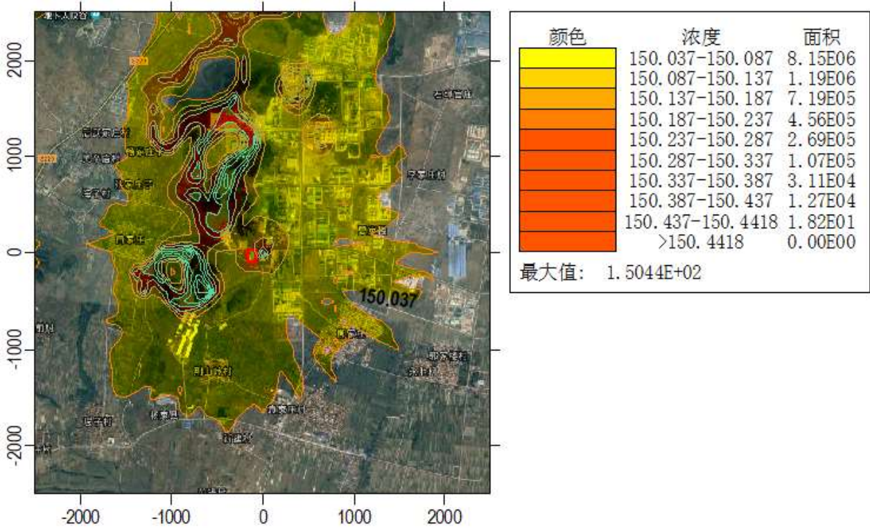
图 5-3 各网格点氨叠加背景值后小时最大平均浓度分布图 单位: \mu\text{g}/\text{m}^3
