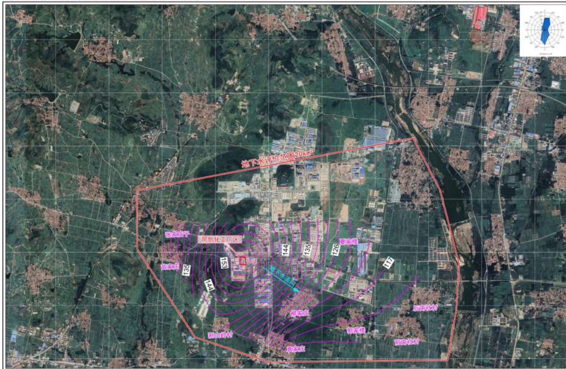
图5-14 地下水等水位线图 比例尺1:40000
