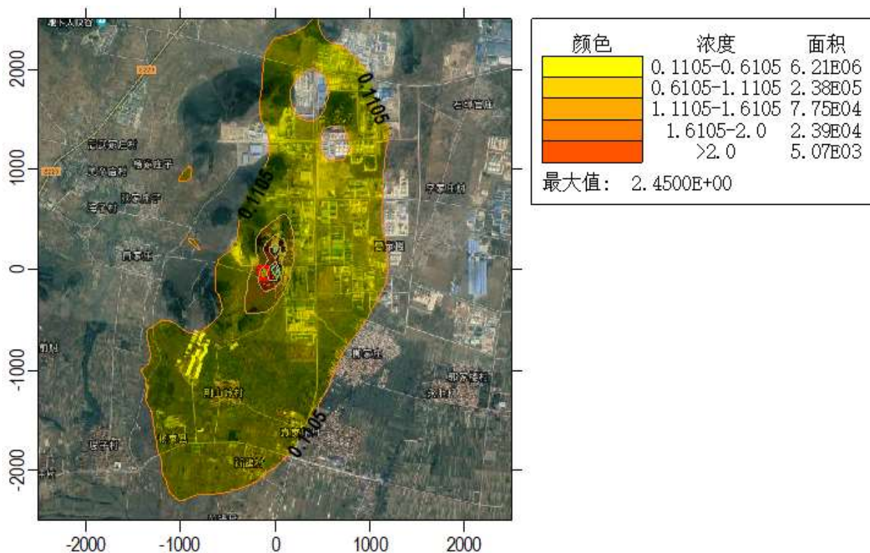
图 5-6 各网格点 PM_{10} 最大年平均浓度分布图 单位: \mu g/m^3
