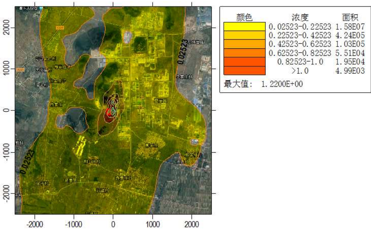
图 5-8 各网格点 PM 2.5 叠加背景值后最大年平均浓度分布图 单位：μg/m 3
