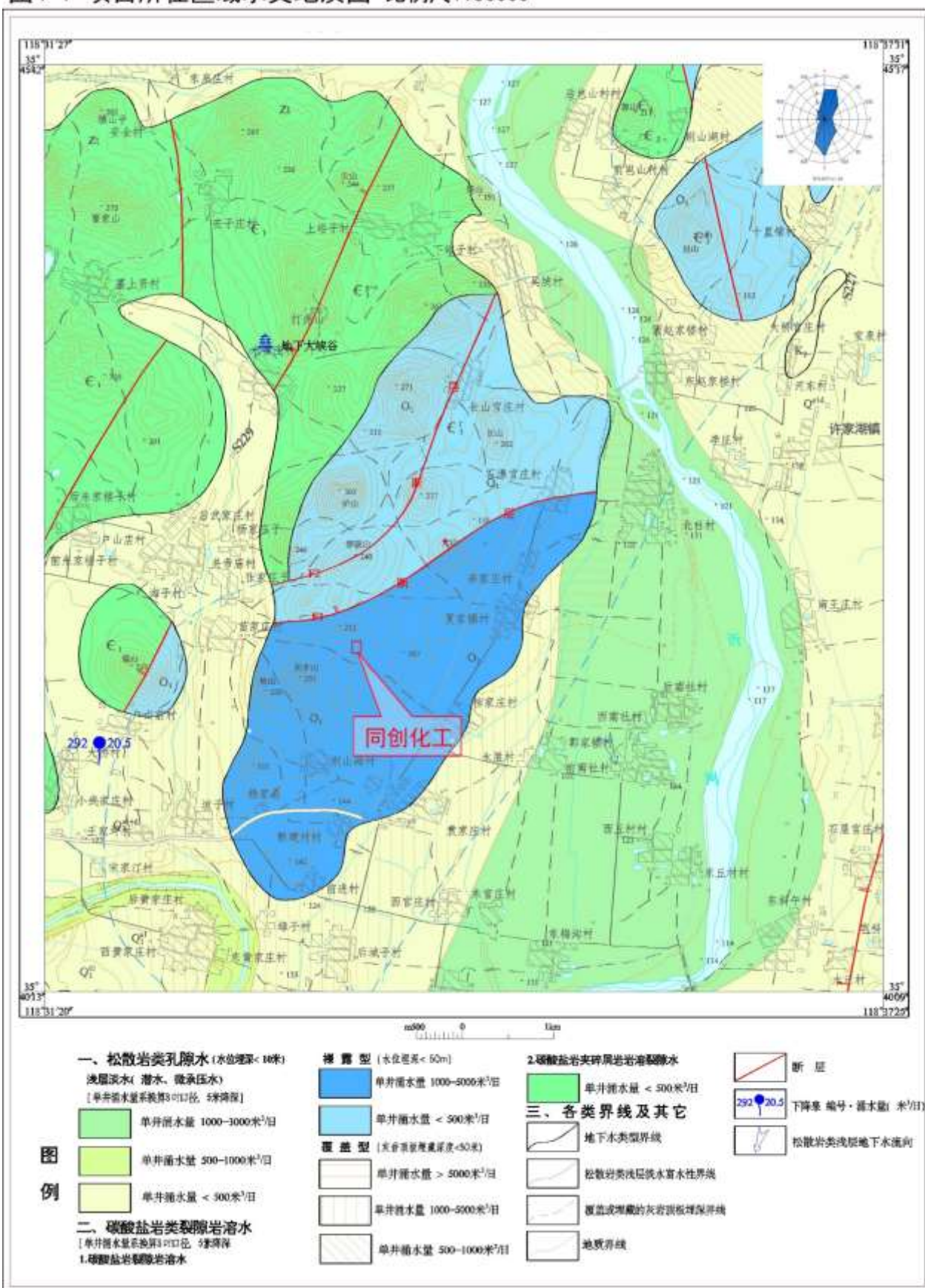
图4-1 项目所在区域水文地质图 比例尺1:50000
