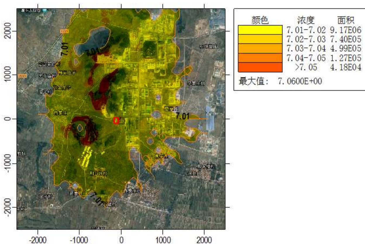
图 5-4 各网格点硫化氢叠加背景值后小时最大平均浓度分布图 单位: \mu\text{g}/\text{m}^3
