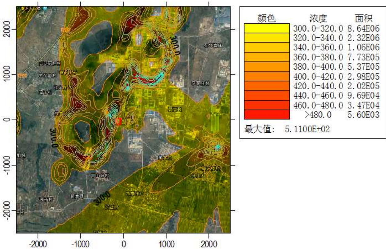
图 5-1 各网格点 VOCs 叠加背景值后小时最大平均浓度分布图 单位：μg/m 3
